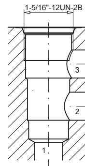
Detaillierte Senkungszeichnung siehe Datenblatt 2.13-1046
