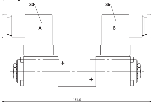
4/3-Wegeventile
