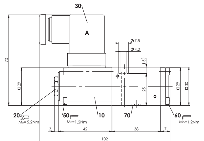
4/2-Wegeventil
